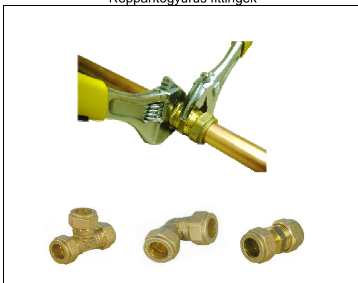
Roppantógyűrűs fittingek
