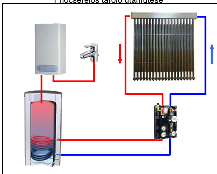
1 hőcserélős tároló utánfűtése
